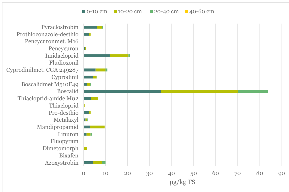
Påviste plantevernmidler og metabolitter i ulike jorddyp for prøver fra skifte med bygg på Haslemoen i 2020.
