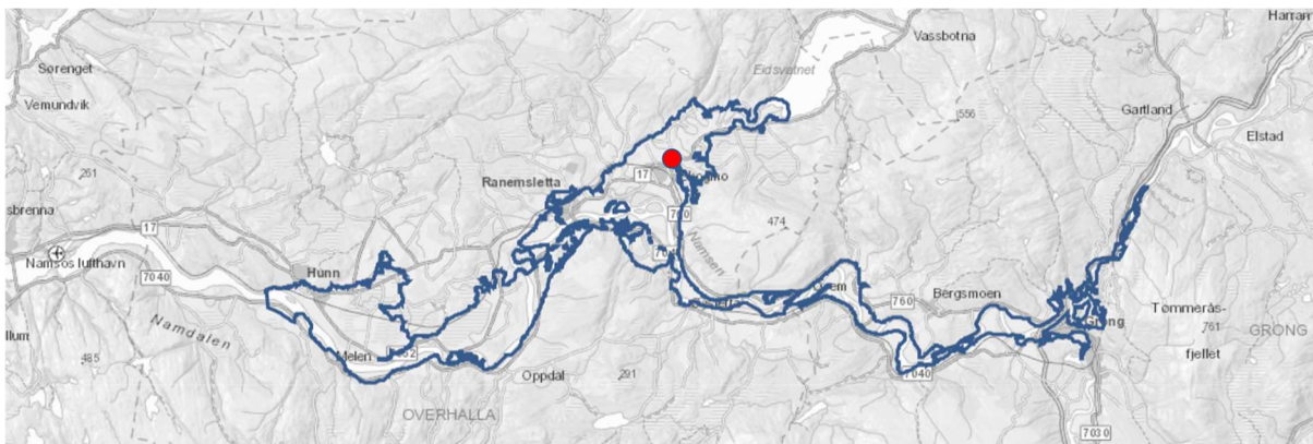
Figur 21. Grunnvannsforkomst 139-864-G Overhalla/Grong. Området for overvåking er markert med rød sirkel.
