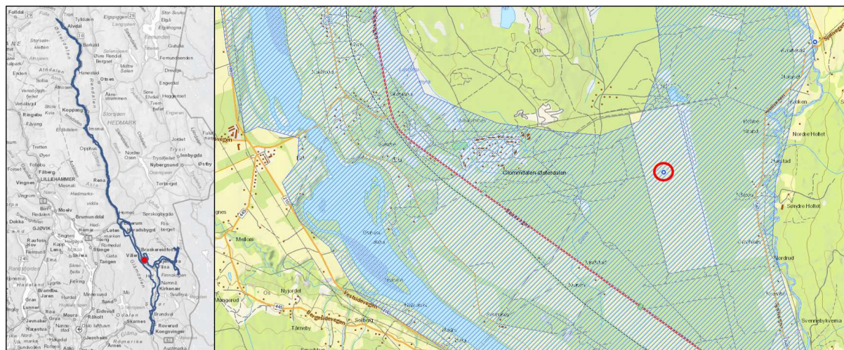
Figur 3. Grunnvannsforekomst 002-724-G Glomdalen-Østerdalen samt plassering av Haslemoen Brønn (VannID- 91946). Fra Vann-Nett og Vannmiljø.
