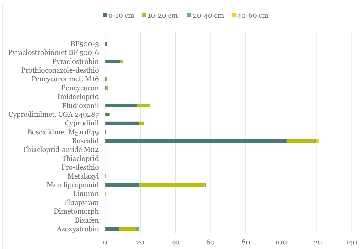
Påviste plantevernmidler og metabolitter i ulike dyp for prøver fra skifte 4 med gulrot på Rimstadmoen 2020.
