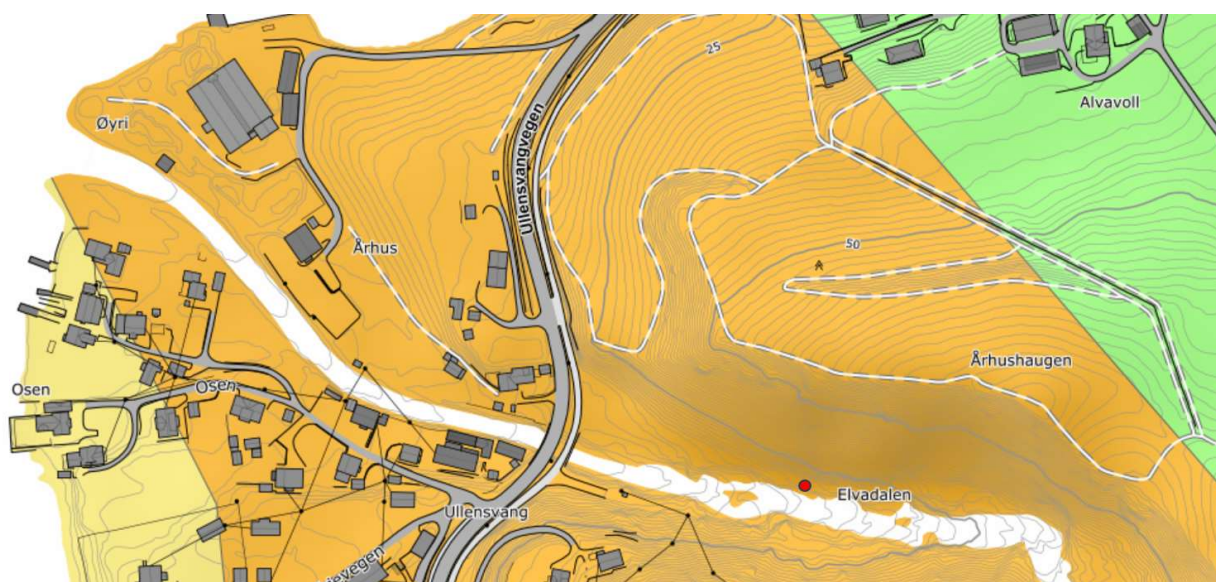
Figur 29. Lofthus Kilde ligger i en større breelvavsetning som også forsyner Lofthus tettsted med kommunalt drikkevann.
