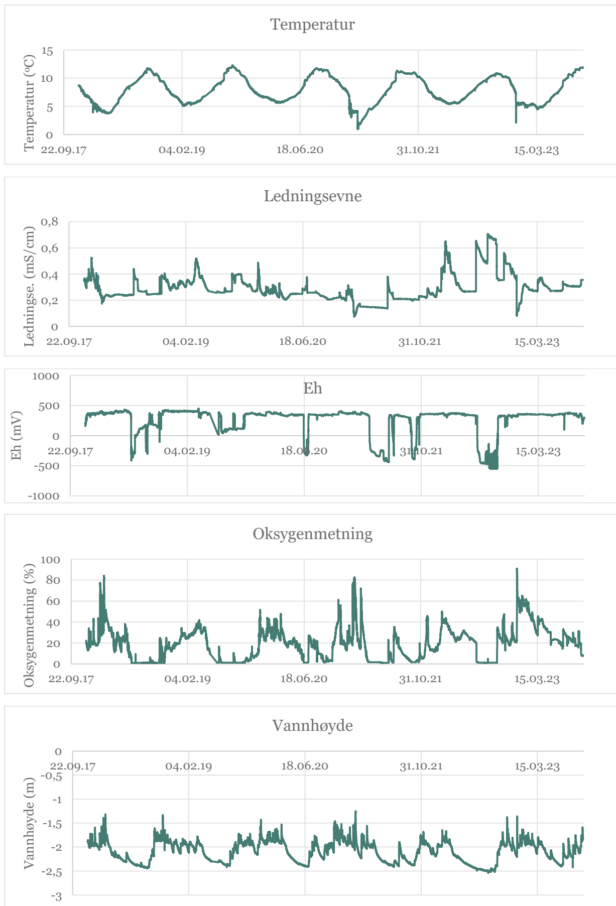
Figur 42. Vannhøyde, oksygen, Eh, ledningsevne og vanntemperatur for Horpestad brønn 25.11.17-27.09.23.
