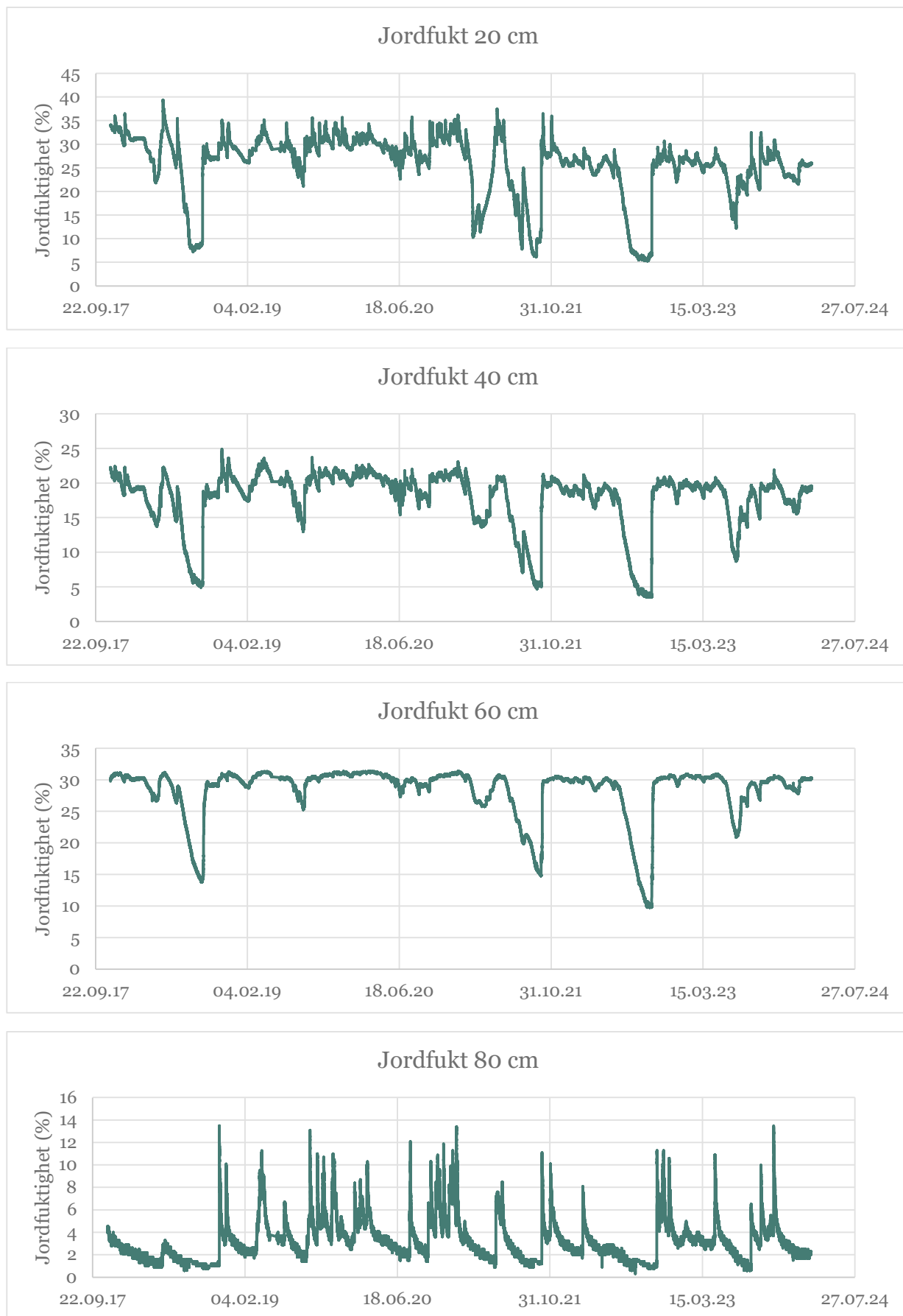
Figur 41. Jordfuktighet ved 20, 40, 60 og 80 cm for jordprofil ved Rimstad kilde 09.11.17-05.03.24
