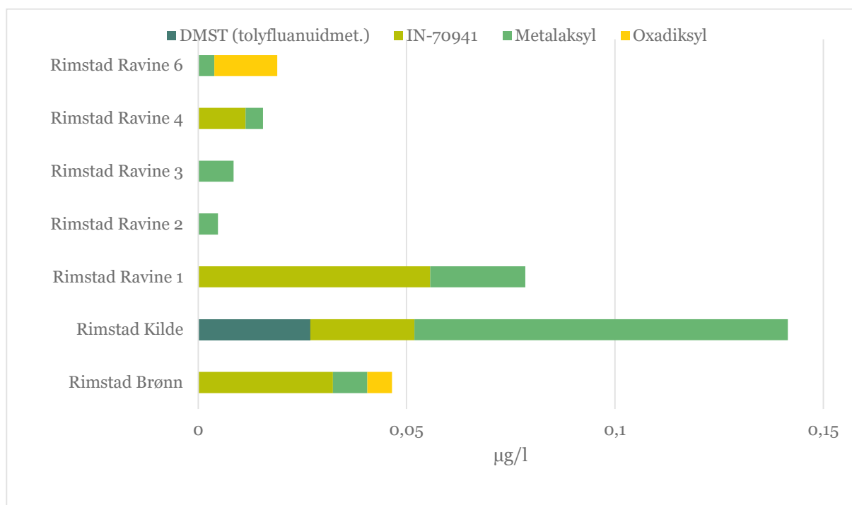
Plantevernmidler og metabolitter påvist i grunnvannskilder i raverer på Rimstadmoen i prøver hentet 11.11.20.
