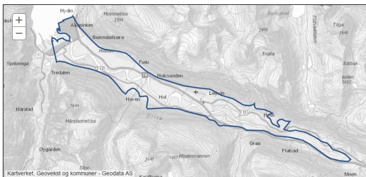
Figur 19. Grunnvannsforekomst 109-678-G Sunndalen. Hentet fra Vann-nett.
