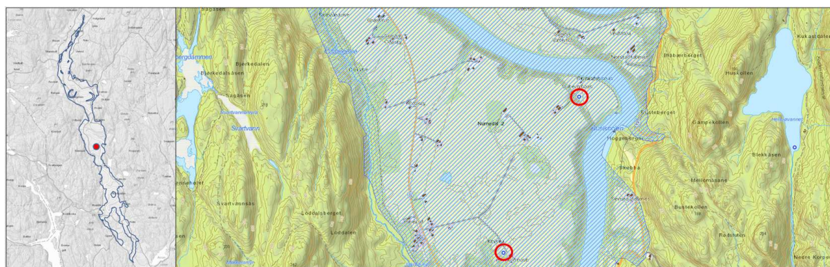
Figur 7. Grunnvannsforekomst 015-746-G Numedal 2, og Rimstad Brønn og Rimstad Kilde. Fra Vann-Nett og Vannmiljø.
