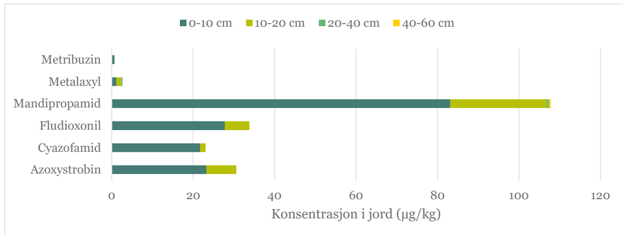
Figur 36. Plantevernmidler påvist i jordprøver fra ulike dyp for potetfelt (Rimstad 1) 14.11.23.
