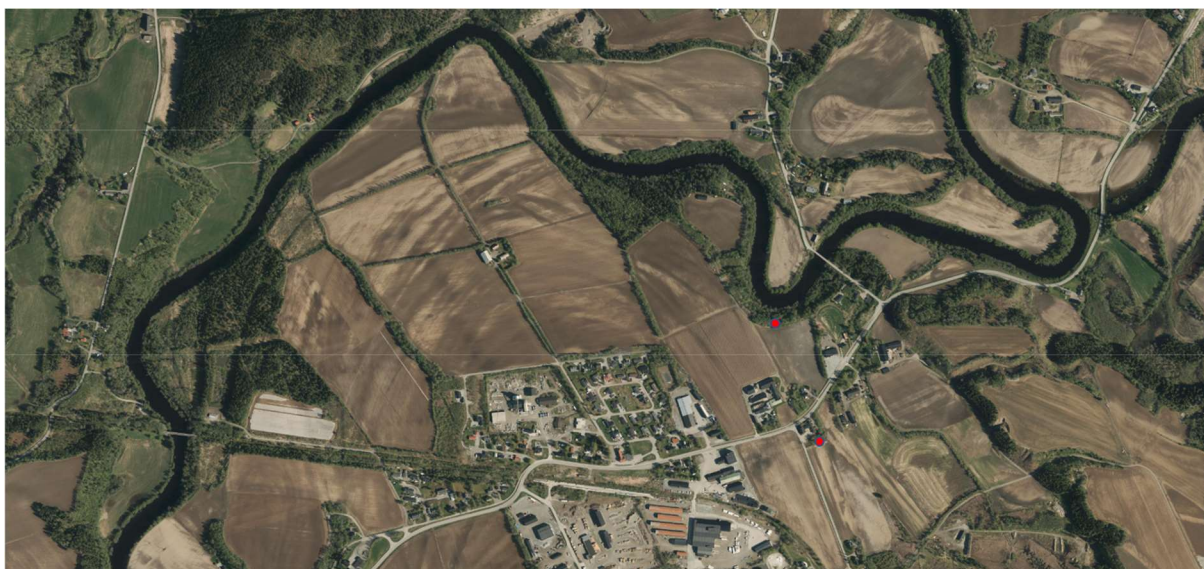
Figur 23. Viser jordbruksarealene rundt Skogmo våren 2020. Røde sirkler markerer kildene som blir undersøkt.
