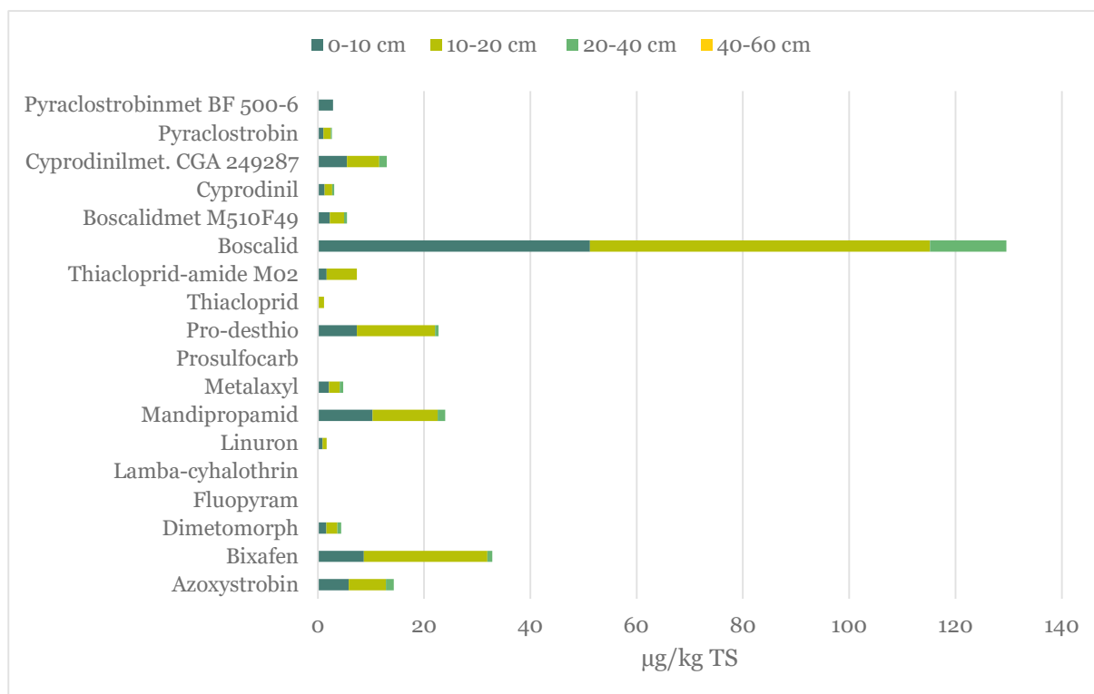
Påviste plantevernmidler og metabolitter i ulike jorddyp for prøver fra skifte med potet på Haslemoen i 2020.
