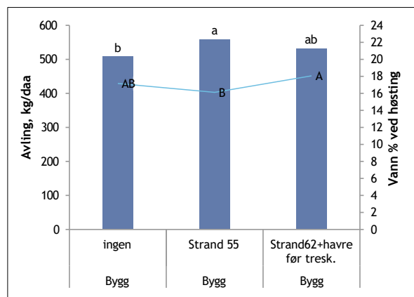
Figur 1. Byggavling (kg/daa) og vann ved høsting (%) i 2021 bygg i reinbestand og tilsådd med fangvekster. Ulike bokstaver viser signifikante forskjeller.
